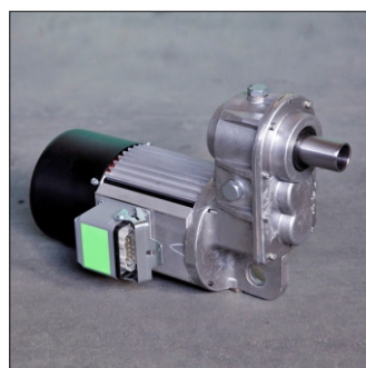
8 Motoréducteur
